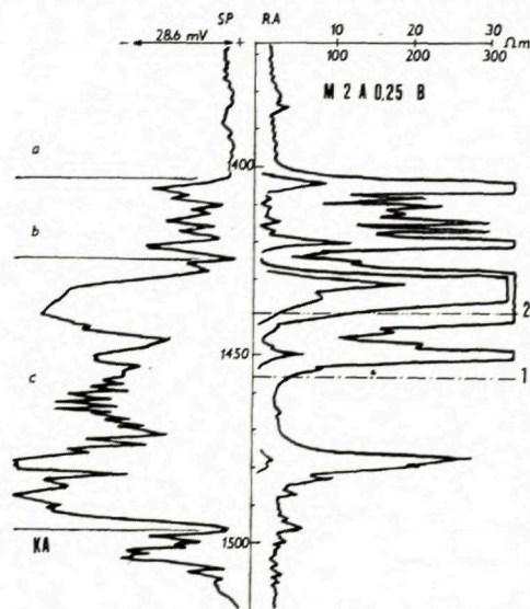
Obr. 48. Elektrokarotážny diagram ropoplynových pieskov stredného badenu vrtu Láb 78. 1 — hranica ropa — voda, 2 — hranica ropa — plyn, a — zóna aglutinancii, b — lábsky obzor, c — lagunárna séria, Ka — karpat, Ra — odporová krivka, SP — krivka vlastných potenciálov
