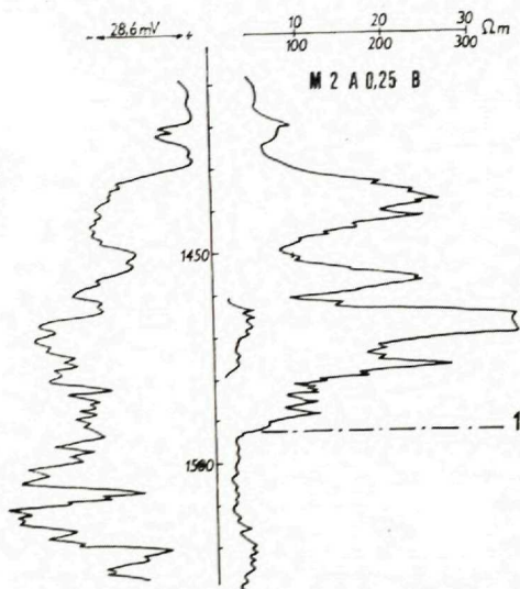
Obr. 64. Elektrokarotážny diagram plynového lábskeho obzoru vrtu Vysoká 21.
