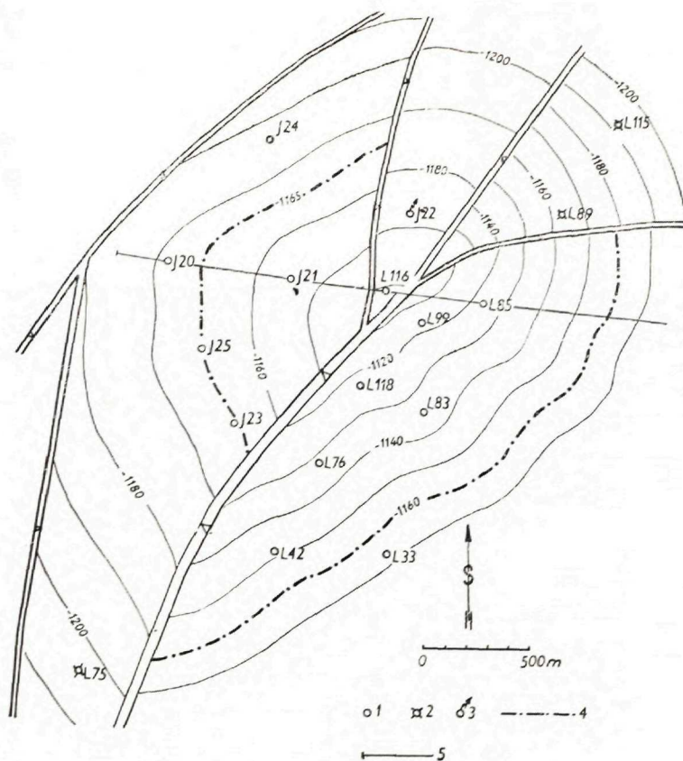
Obr. 50. Štruktúrna mapa povrchu vrchnobaden-ského plynového obzoru 1 — plynová sonda, 2 — negatívny vrt, 3 — erup-tovaný vrt, 4 — hranica plyn — voda, 5 — geo-logický rez (obr. 46)
