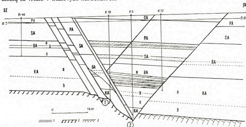
Obr. 29. Priechy geologický rez neogénom ložiska Kúty.
