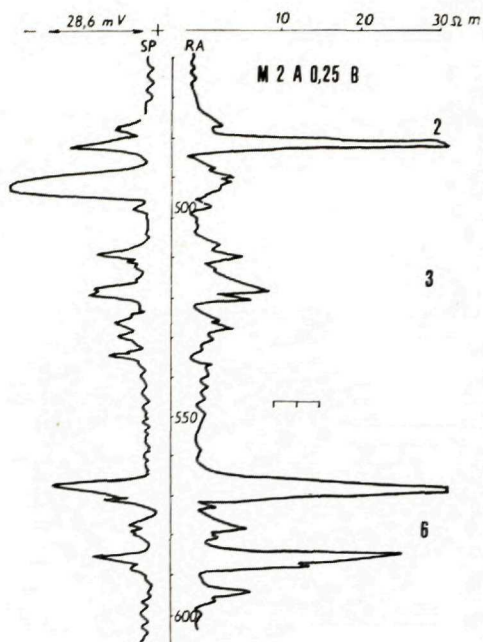
Obr. 37. Elektrokarotážny diagram sarmatských plynových obzorov vrtu Studienka 44.
