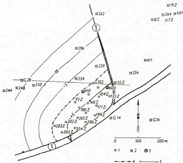
Obr. 9. Cigánske pole. Štruktúrna mapa povrchu sarmatského roponosného obzoru. 1 — pozitívny vrt, 2 — negatívny vrt, 3 — objavné vrty, 4 — hranica ropa — voda, 5 — geologický rez (obr. 2), 1 — severný farský zlom, 2 — zlom Cigánskeho poľa
