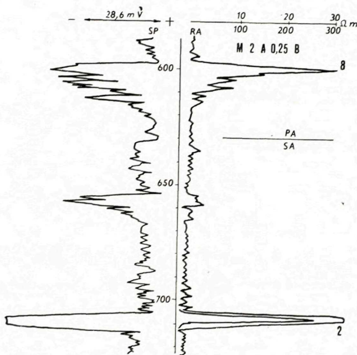
Obr. 58. Elektrokarotážny diagram plynových obzorov vrtu Jakubov 4. 1 — vodonosný obzor, 2 — sarmatský plynový obzor, 8 — panónsky plynový obzor PA/SA — hranica panón—sarmat, Ra — odporová krivka, SP — krivka vlastných potenciálov
