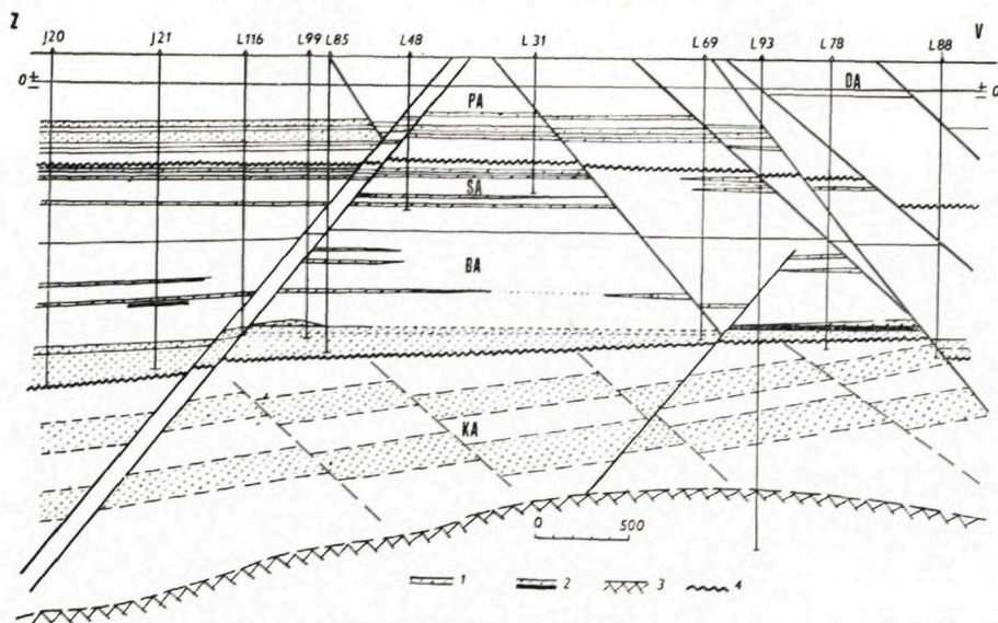
Obr. 46. Priechový geologický rez neogénom ložiska Láb.
