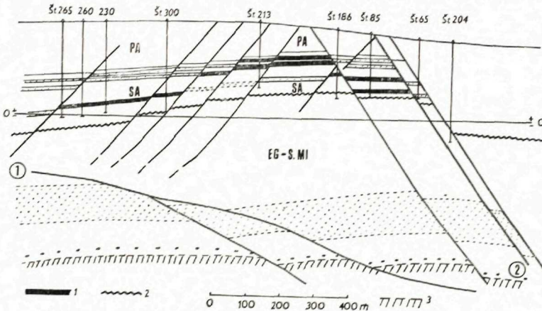
Obr. 11. Priečný geologický rez neogénom ložiska Štefanov.
