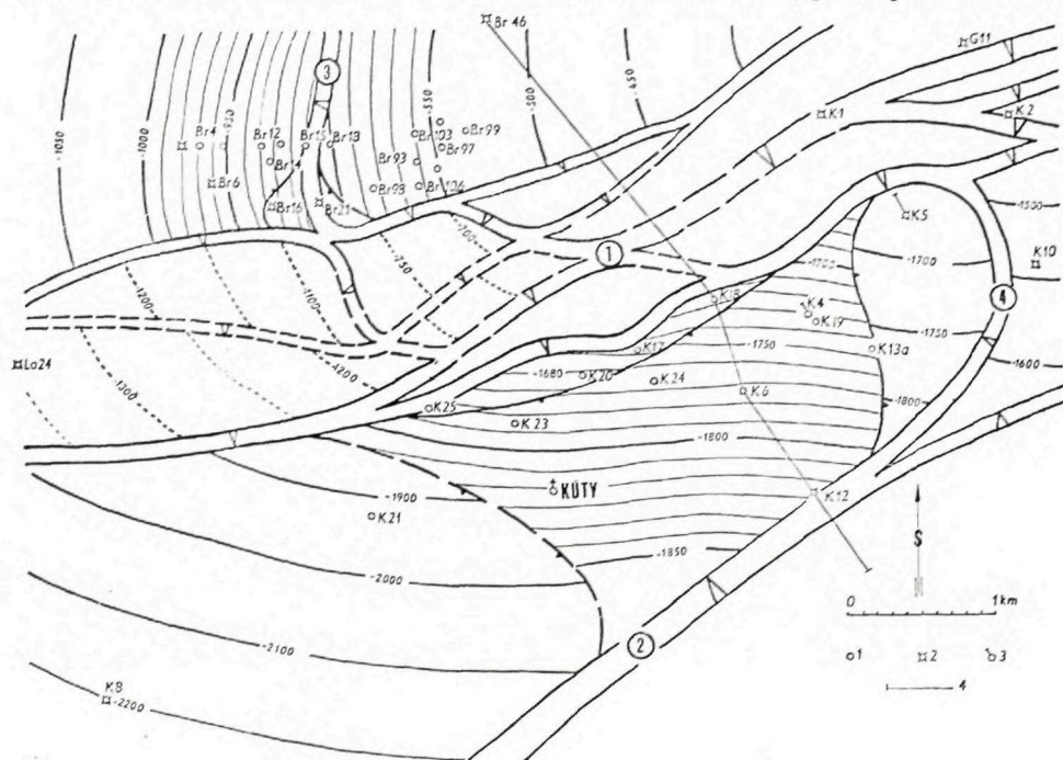
Obr. 30. Ložisko Kútý. Štruktúrna mapa povrchu 2. badenského obzoru.
