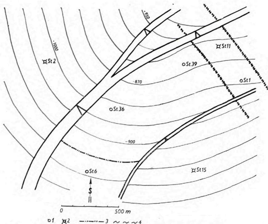
Obr. 38. Štruktúrna mapa povrchu vrchnobadenského plynového obzoru.
