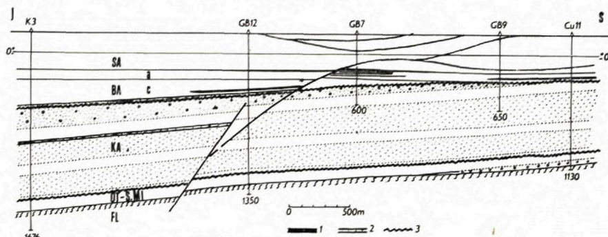
Obr. 21. Pozdĺžny geologický rez neogénom ložiska B-pole.
