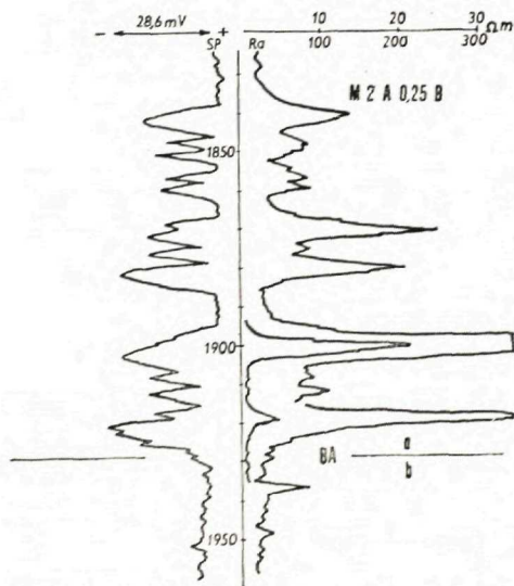
Obr. 31. Elektrokarotážny diagram vrchnobadenských plynových obzorov vrtu Kúty 20. Ra — odporová krivka, SP — krivka vlastných potenciálov, BA — baden, a — vrchný baden b — stredný baden
