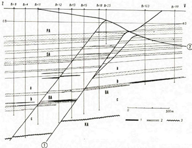
Obr. 25. Priečný geologický rez neogénom ložiska Brodské.
