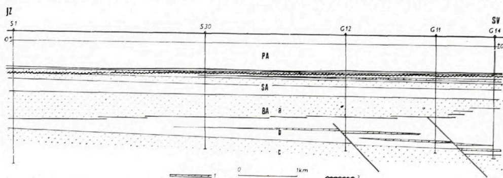
Obr. 59. Pozdĺžny geologický rez panónom, sarmatom a badenom ložiska Suchohrad — Gajary. 1 — plyn, 2 — diskordancia, PA — panón, SA — sarmat, BA — baden, a — vrchný baden, b — stredný baden, c — spodný baden
