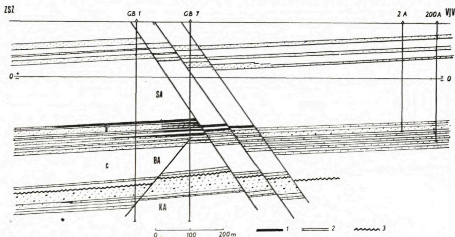
Obr. 23. Priečný geologický rez strednou časťou ložiska B-pole.
