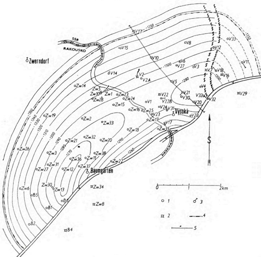
Obr. 63. Ložisko Vysoká — Zwerndorf. Štruktúrna mapa povrchu lábskeho obzoru. 1 — plynová sonda, 2 — negatívny vrt, 3 — odklonený vrt, 4 — hranica plyn — voda, 5 — geologický rez (obr. 62)
