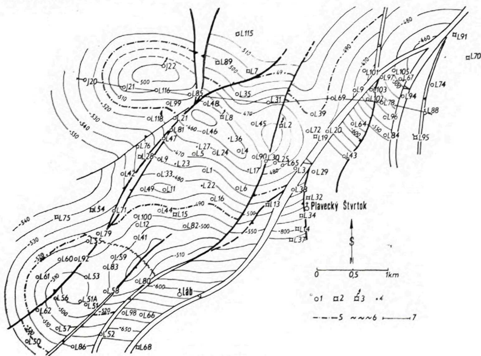
Obr. 52. Štruktúrna mapa povrchu 2. sarmatského obzoru.
