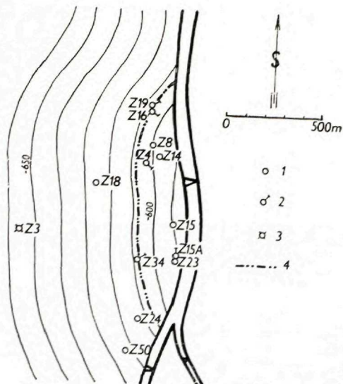
Obr. 42. Štruktúrna mapa povrchu vrchnobadenského plynového obzoru.
