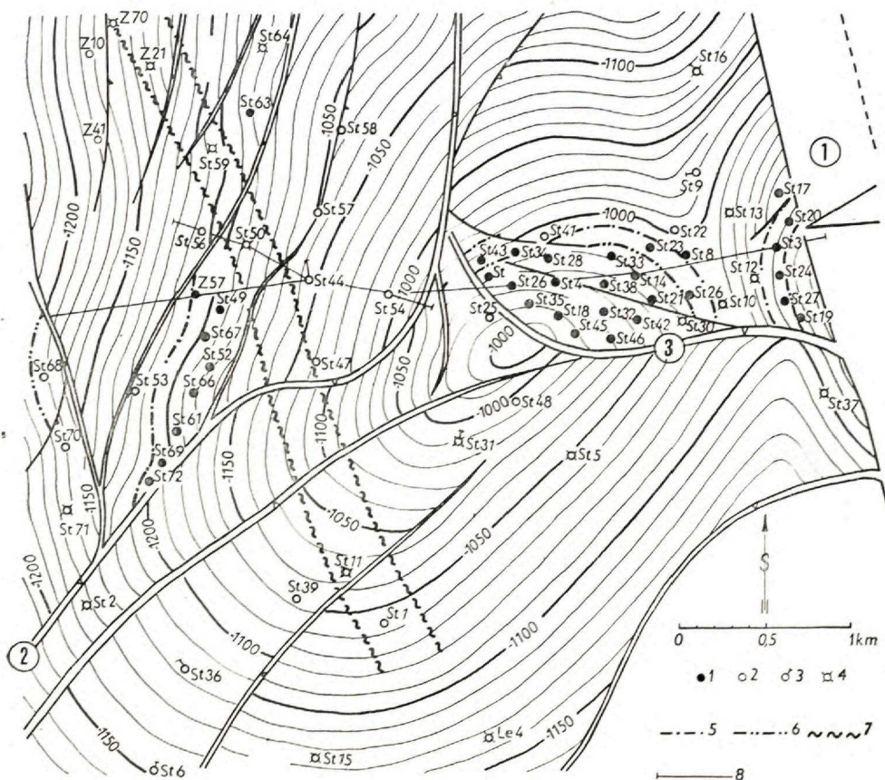
Obr. 33. Ložisko Studienka. Štruktúrna mapa povrchu lábskeho obzoru.
