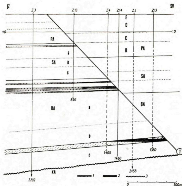
Obr. 39. Priečný geologický rez neogénom ložiska Závod. 1 — plyn, 2 — ropa, 3 — diskordancia, 1 — závodský zlom, PA — panón, B, C, D, E — zóny panónu, SA — sarmat, a — vrchný sarmat, b — stredný sarmat, c — spodný sarmat, BA — baden, a — vrchný baden, b — stredný baden, c — spodný baden, KA — karpát
