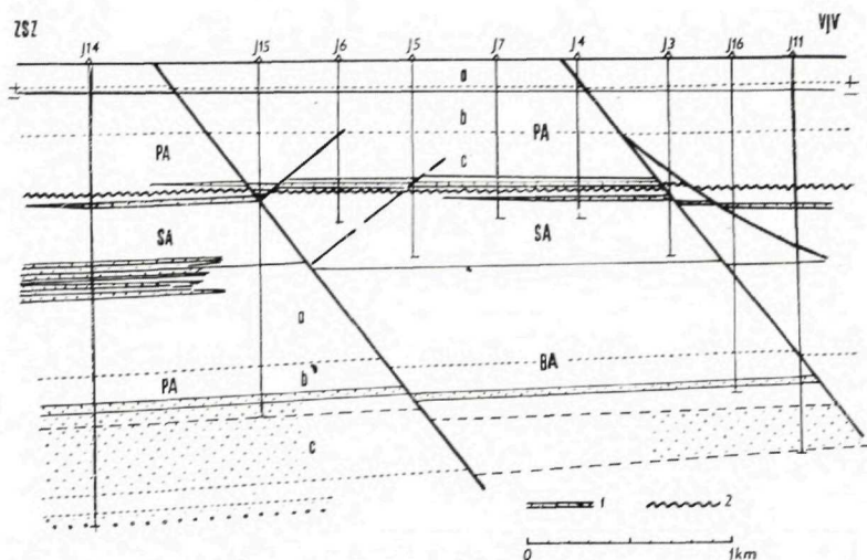
Obr. 56. Geologický rez panónom, sarmatom a badenom ložiska Jakubov. 1 — plyn, 2 — diskordancia, PA — panón, a — vrchný panón, b — stredný panón, c — spodný panón, SA — sarmat, BA — baden, a — vrchný baden, b — stredný baden, c — spodný baden
