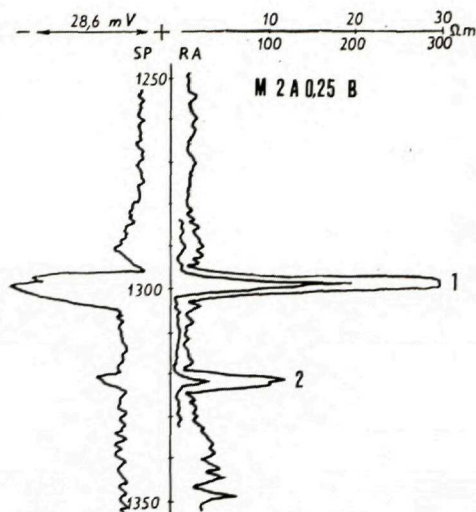
Obr. 34. Elektrokarotážny diagram roponosného lábskeho obzoru a plynového obzoru lagunárnej série vrtu Studienka 61.
