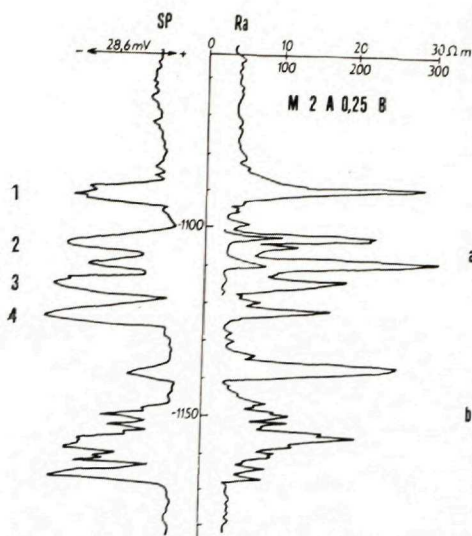
Obr. 41. Elektrokarotážny diagram roponosných pieskov lábskeho obzoru vrtu Závod 20. 1—4 — roponosný piesok, a — lábsky obzor, b — lagunárna séria, Ra — odporová krivka, SP — krivka vlastných potenciálov
