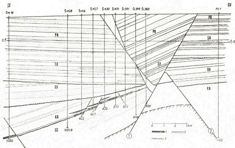
Obr. 14. Priečný geologický rez neogénom ložiska Petrova Ves.
