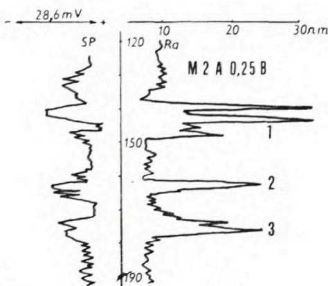
Obr. 8. Elektrokarotážny diagram sarmatského roponosného obzoru vrtu Gbely 27.
