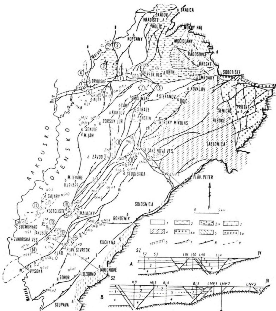
Obr. 1. Odkrytá tektonická mapa a priečne geologické rezy slovenskej časti viedenskej panvy.
