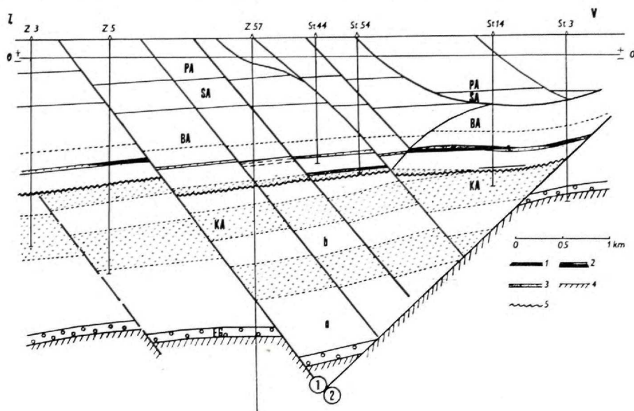
Obr. 32. Priečný geologický rez neogénom ložísk Závod — Studienka.
