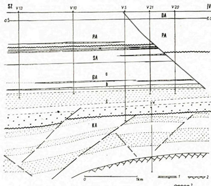
Obr. 62. Geologický rez neogénom ložiska Vysoká — Zwerndorf.
