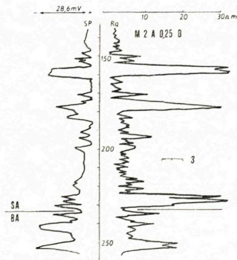
Obr. 4. Elektrokarotážny diagram sarmatských roponosných obzorov vrtu Gbely 70.
