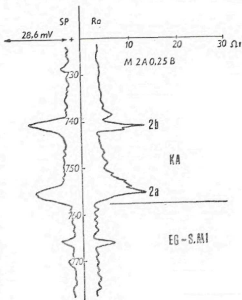
Obr. 16. Elektrokarotážny diagram karpatských roponosných obzorov vrtu Štefanov 428.
