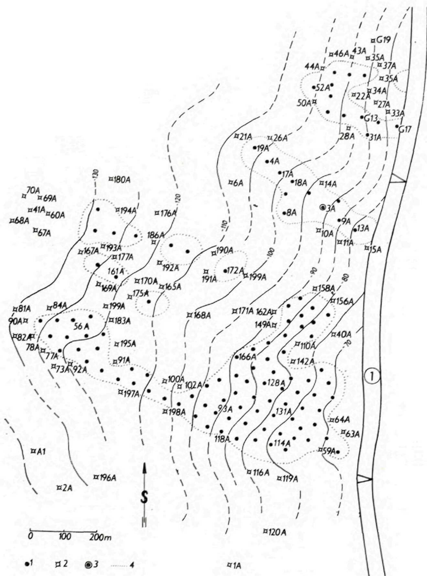
Obr. 5. A-pole. Štruktúrna mapa povrchu roponosného obzoru.
