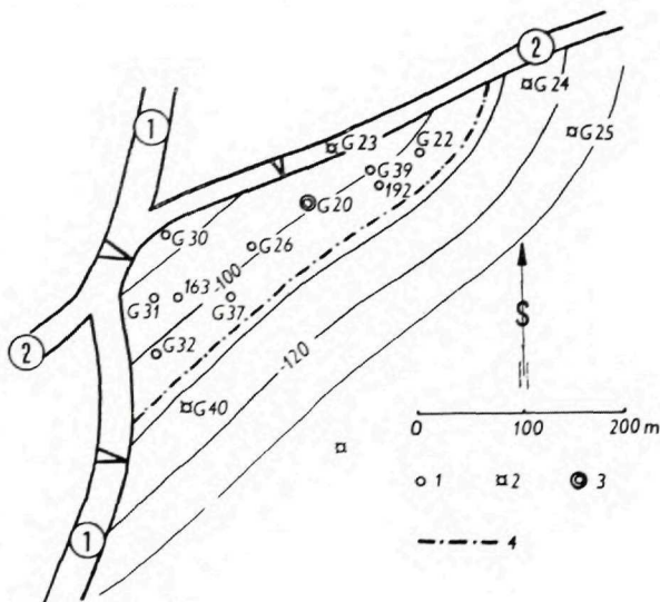
Obr.10. Farské pole. Štruktúrna mapa povrchu roponosného obzoru.
