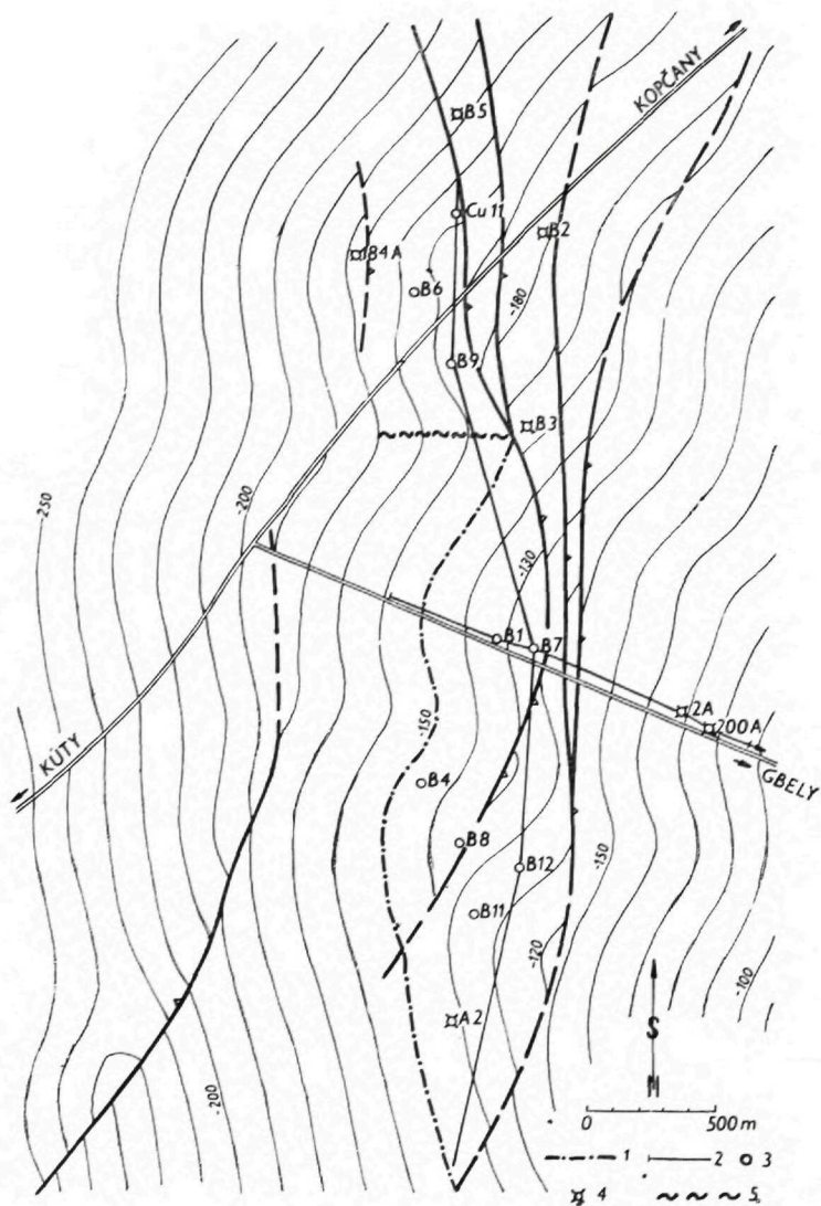
Obr. 22. Ložisko B-pole. Štruktúrna mapa povrchu 1. vrchnobadenského obzoru.
