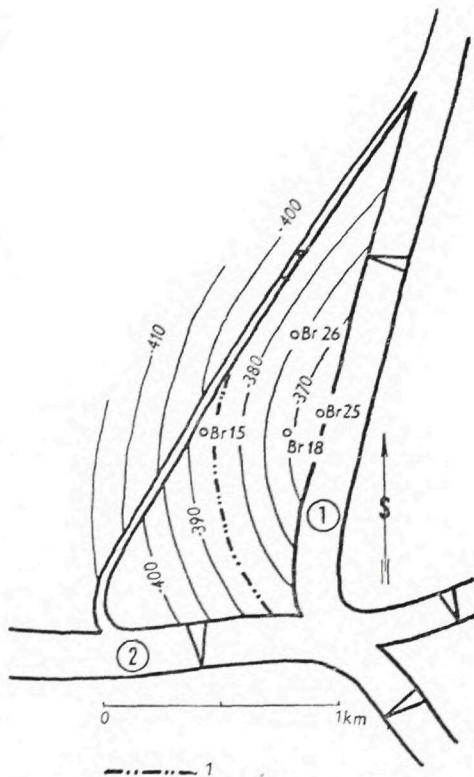
Obr. 28. Štruktúrna mapa povrchu sarmatského plynového obzoru.
