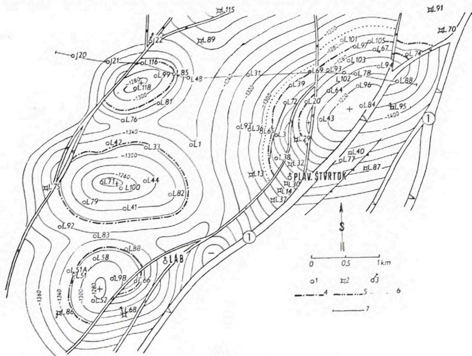
Obr. 47. Ložisko Láb. Štruktúrna mapa povrchu lábskeho obzoru a litavských vápencov.
