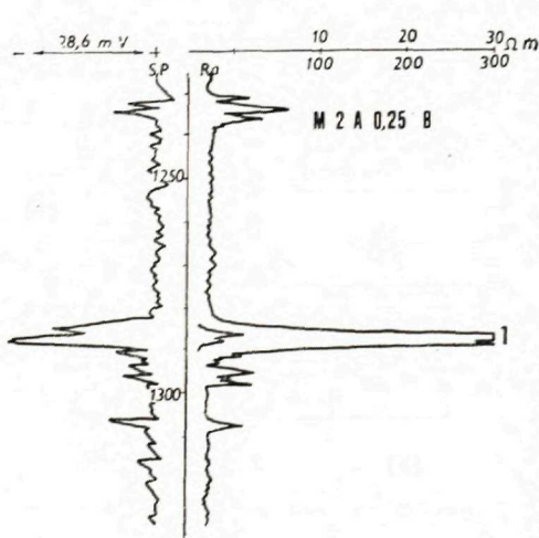
Obr. 51. Elektrokarotážny diagram vrchnoba-denského plynového obzoru vrtu Láb 76.
