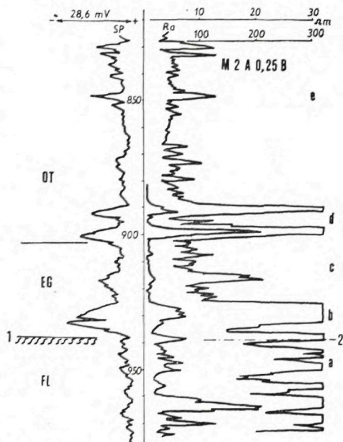
Obr. 20. Elektrokarotážny diagram roponosných obzorov vrtu Cunín 20.
