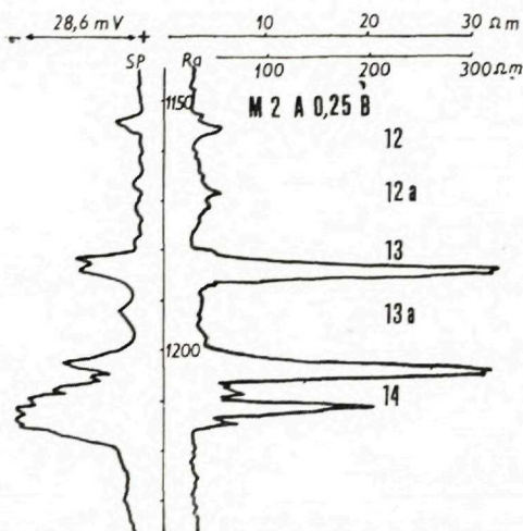
Obr. 27. Elektrokarotážny diagram roponosných pieskov vrtu Brodské 39.
