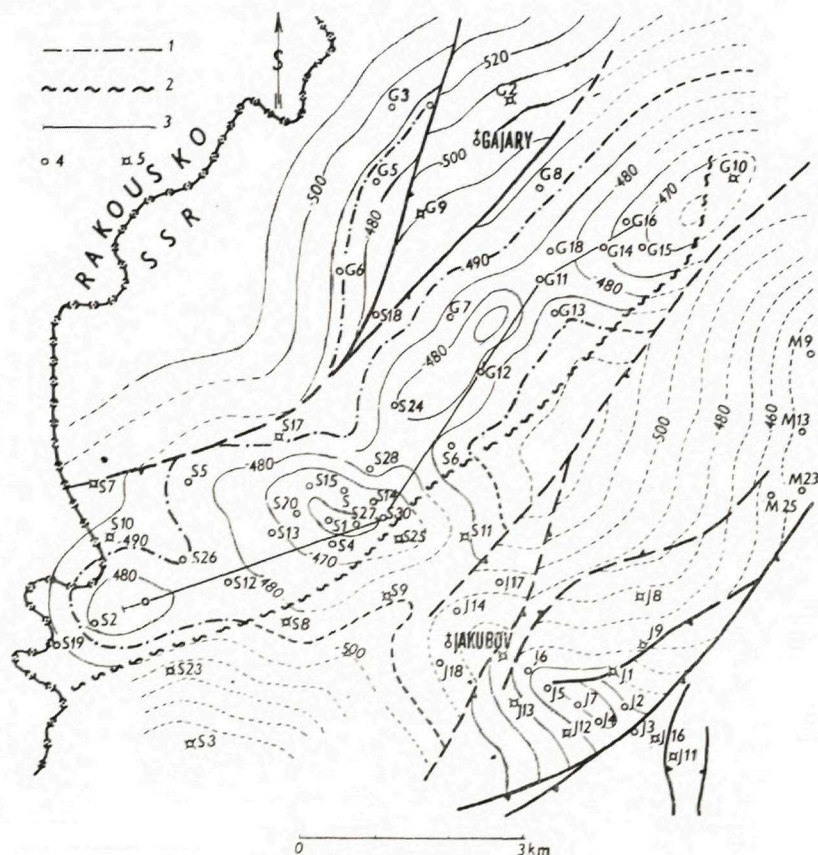
Obr. 60. Ložisko Suchohrad — Gajary. Štruktúrna mapa povrchu panónskeho plynového obzoru.
