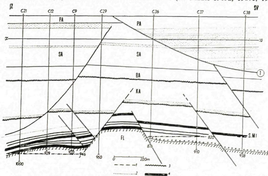
Obr. 17. Pričný geologický rez neogénom ložiska Cunín.
