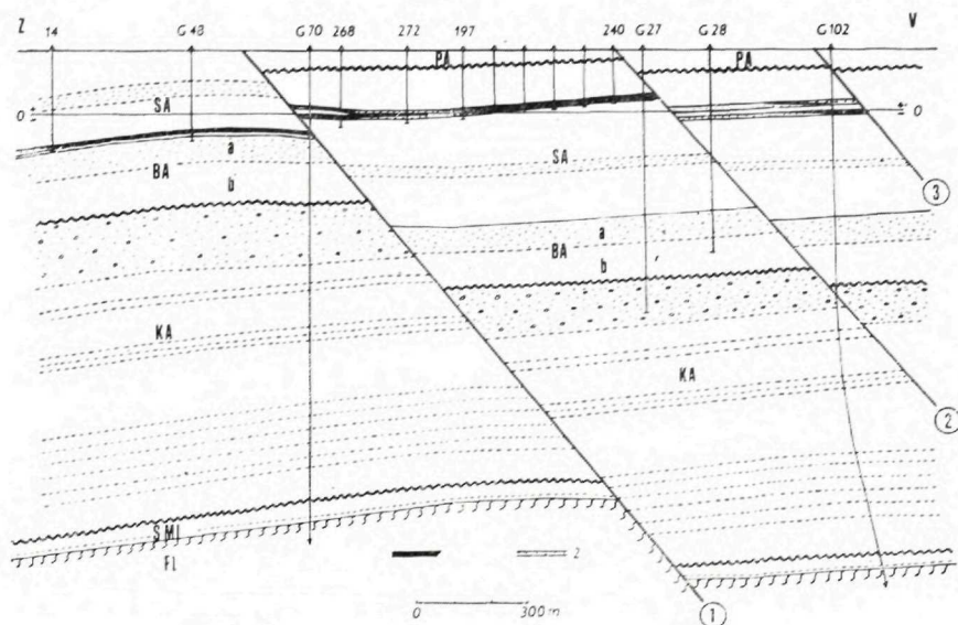
Obr. 2. Geologický rez neogénom ložísk Starého, Nového a Cigánskeho poľa. 1 — ropa, 2 — plyn, 1 — gbelsko-hodonínsky zlom 2 — zlom Nového poľa, 3 — zlom Cigánskeho poľa, PA — panón, SA — sarmat, BA — baden, a — vrchný baden, b — spodný baden, KA — karpat, SMI — spodný miocén, FL — flyš Abb. 2. Geologischer Schnitt durch das Neogen der Lagerstätten Altfeld, Neufeld und Zigeunerfeld. 1 — Erdöl, 2 — Erdgas, 1 — Gbely—Hodonin Bruch, 2 — Neufeldsbruch, 3 — Zigeunerfeldsbruch, PA — Pannon, SA — Sarmat, BA — Baden, a — Oberbaden, b — Unterbaden, KA — Karpat, SM — Untermiozän, FL — Flysch
