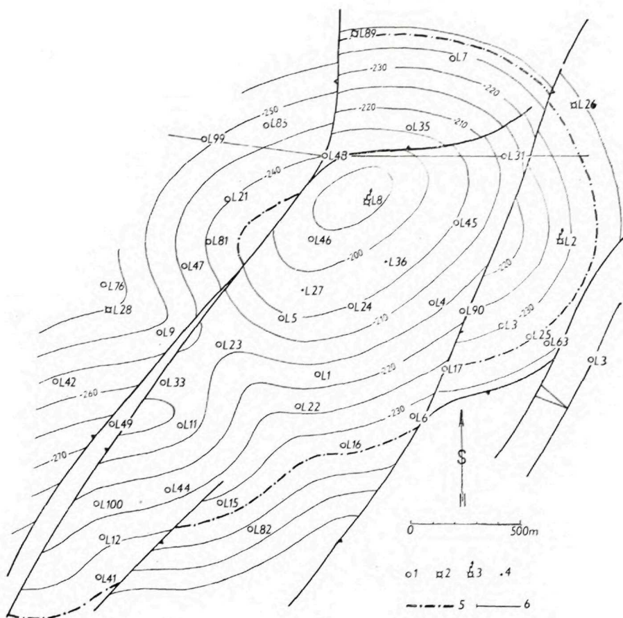
▲ Obr. 54. Štruktúrna mapa povrchu 6. panónskeho plynového obzoru.
