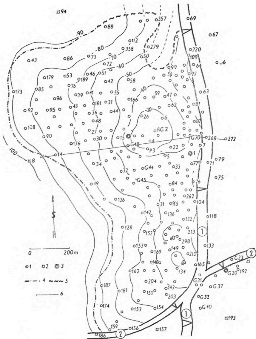
Obr. 3. Staré pole. Štruktúrna mapa povrchu roponosného obzoru. 1—pozitívny vrt, 2—negatívny vrt, 3—objavné vrty, 4—hranica ropa—voda, 5—hranica vyklinenia, 6—geologický rez (obr. 2), 1—gbelsko-hodonínsky zlom, 2—severný farský zlom.
