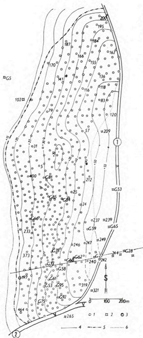
Obr. 7. Nové pole. Štruktúrna mapa povrchu sarmatského roponosného obzoru.
