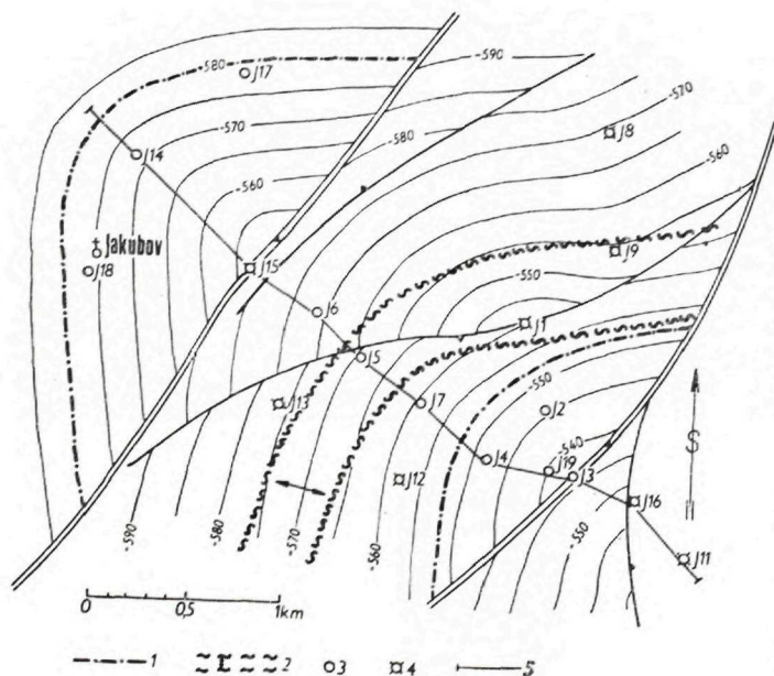
Obr. 57. Ložisko Jakubov. Štruktúrna mapa povrchu 2. sarmatského obzoru.
