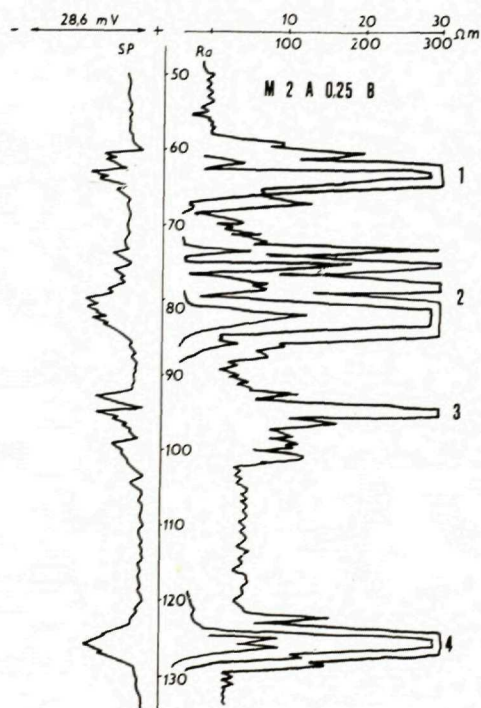
Obr. 13. Elektrokarotážny diagram sarmatských roponosných obzorov.
