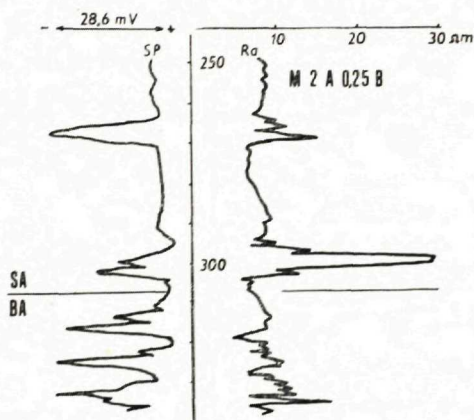
Obr. 6. Elektrokarotážny diagram sarmatského roponosného obzoru vrtu 161A.
